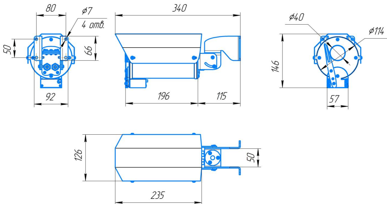
Рисунок 1 – общий вид, габаритные и присоединительные размеры
